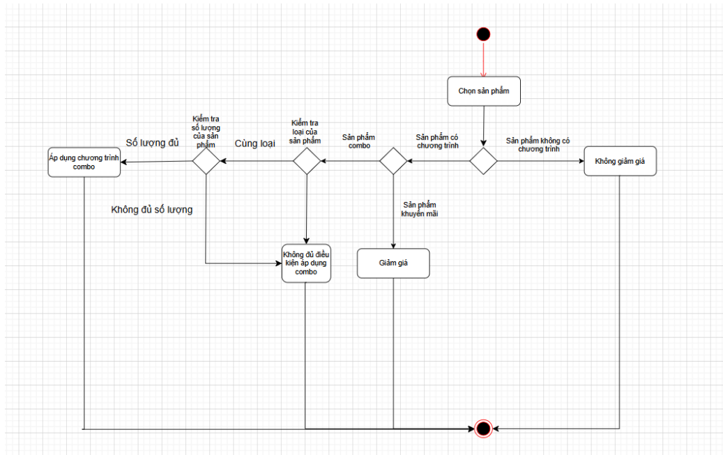
Ảnh 5. Activities diagram cho combo- sửa lại các điều kiện so sánh sản phẩm.
