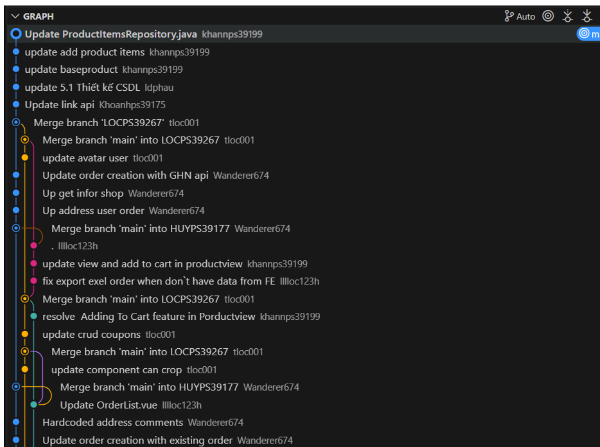
Ảnh 35. Quản lý trong việc trên GitHub.
