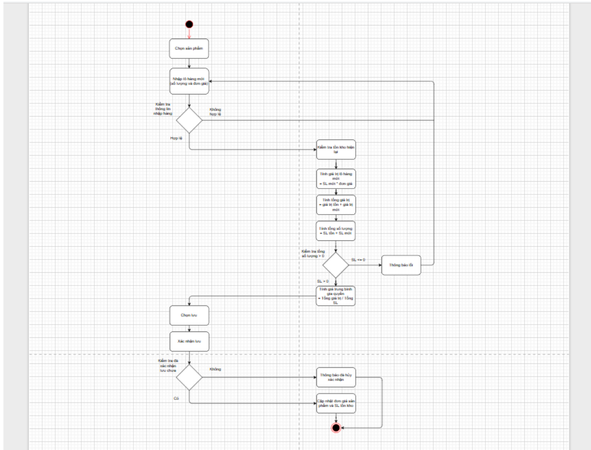
Ảnh 2. Activities diagram cho tính bình quân gia quyền giá sản phẩm.
